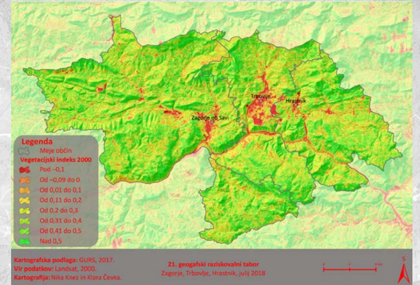
NDVI leta 2000
