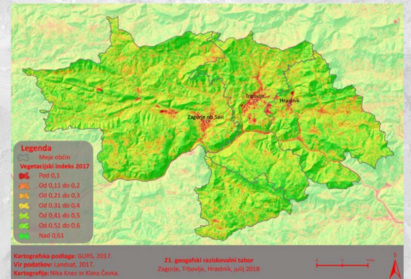
NDVI leta 2017
